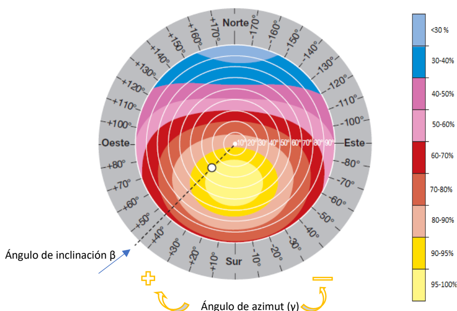
Figura 55. Porcentaje de energía respecto al máximo como consecuencia de las pérdidas por orientación e inclinación. Fuente: ABB, 2011
