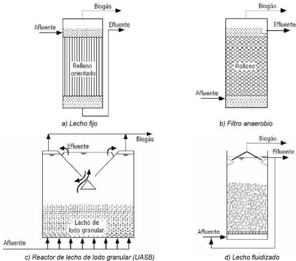
Figura 24. Esquema de reactores con retención interior de biomasa. Fuente: IDAE, 2007
