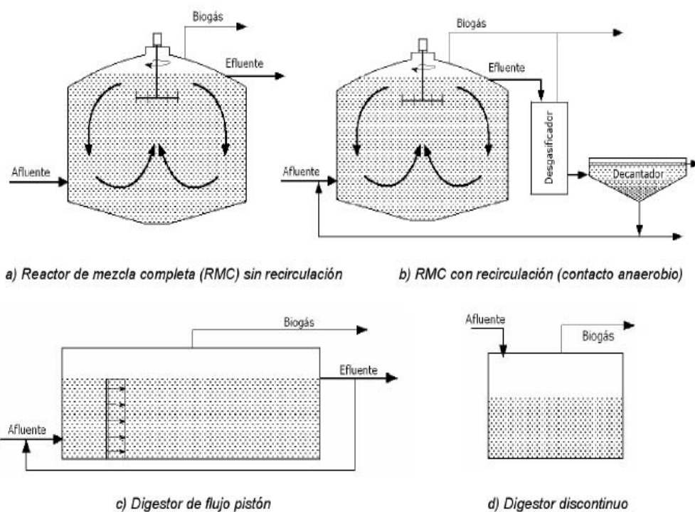
Figura 23. Esquema de reactores sin retención interior de biomasa. Fuente: IDAE, 2007.
