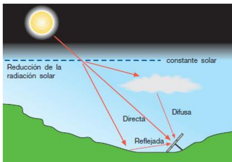
Figura 40. Componentes de la radiación solar. Fuente: ABB, 2011
