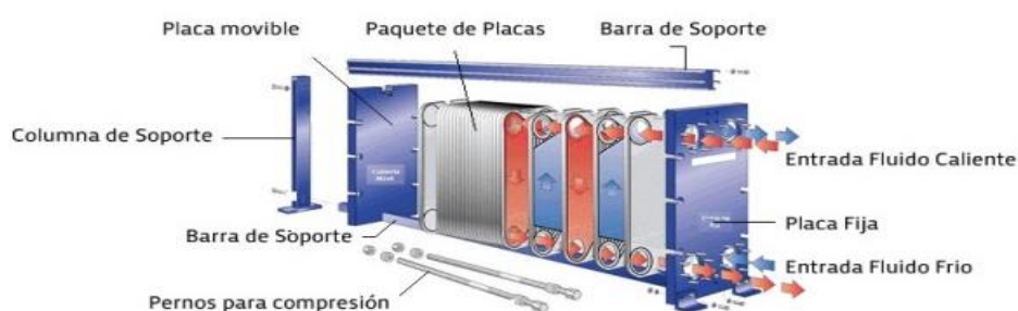
Figura 67. Partes de un intercambiador de placas. Fuente: www.saincal.com
