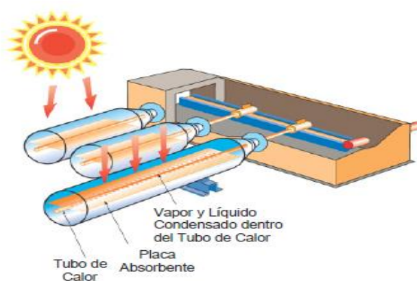
Figura 64. Colector de tubo de vacío. Fuente: Garwood, 2005.
