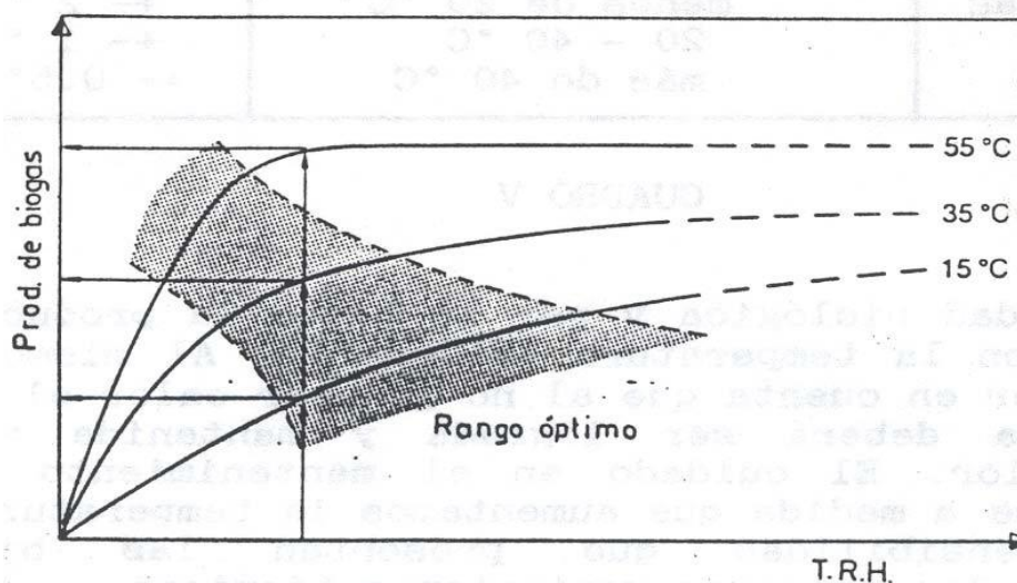
Figura 35. Relación TRH -producción de biogás. Fuente: Hillbert, 2003
