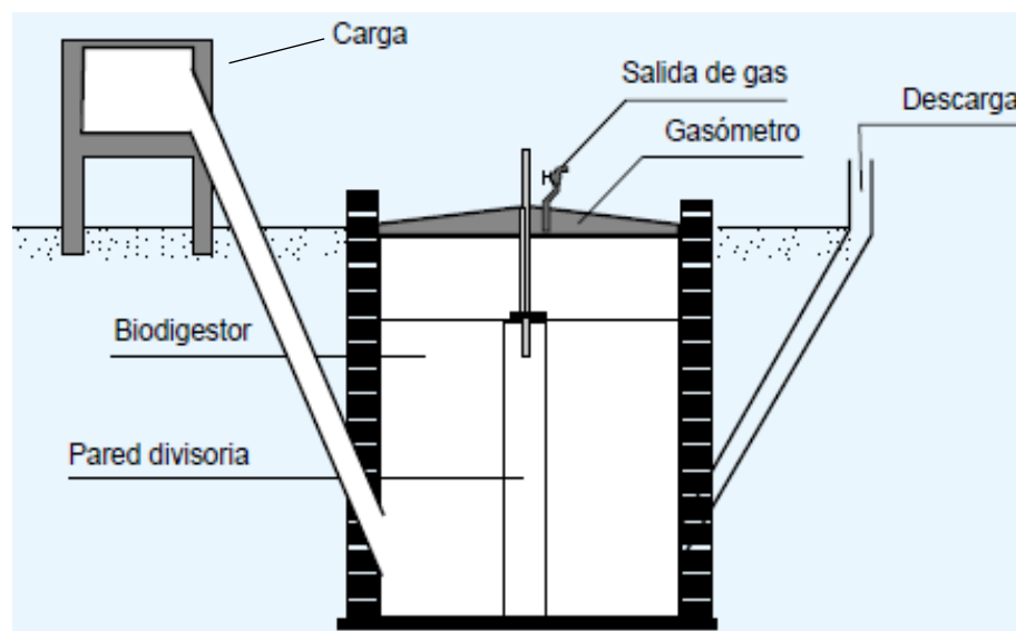
Figura 32. Digestor tipo hindú. Fuente: Varnero, 2011
