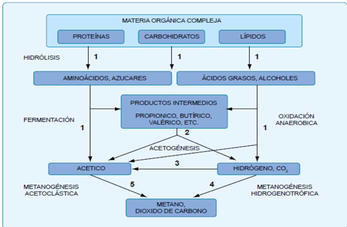
Figura 22. Esquema de reacciones de la digestión anaeróbica. Fuente: Gobierno de Chile
