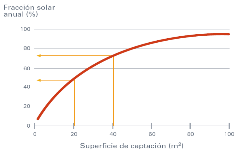
Figura 78. Variación de la fracción solar con la superficie de captación. Fuente: Belso, 2011.
