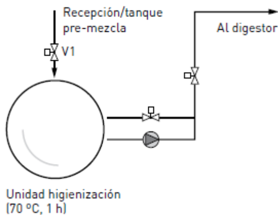
Figura 37. Diagrama de flujo pretratamiento térmico: pasteurización. Fuente: IDAE, 2011
