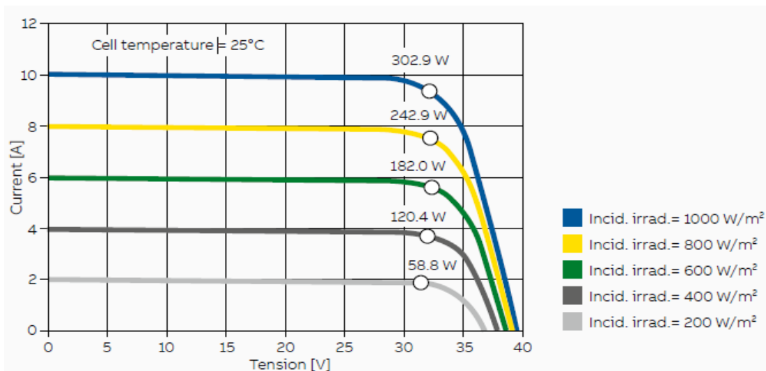
Figura 57. Curva característica V-I de la célula FV en función de la irradiancia incidente. Fuente: ABB, 2019.
