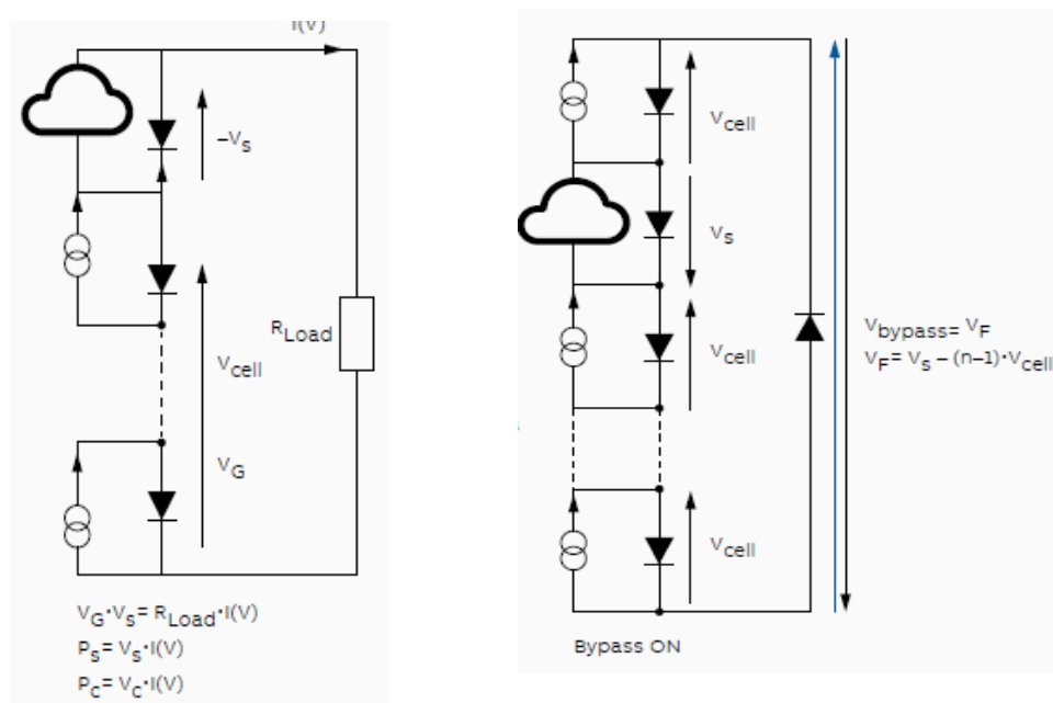
Figura 59. esquema comparativo módulo FV sin y con bypass. Fuente: ABB, 2019.
