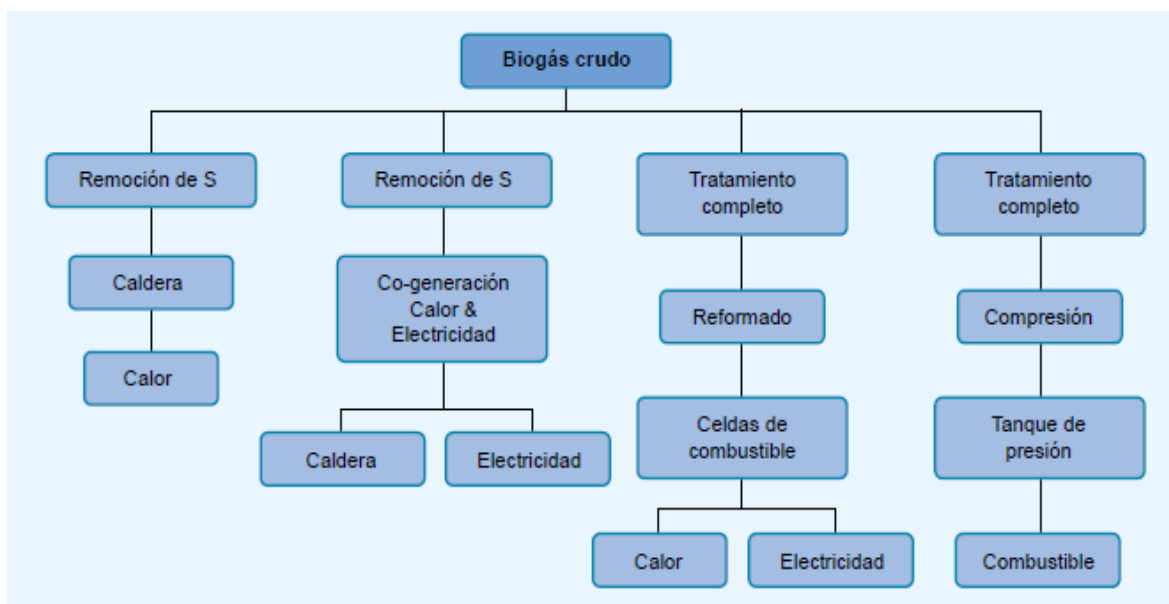
Figura 39. Alternativas de utilización del biogás y sus requerimientos de purificación. Fuente: Varnero, 2011
