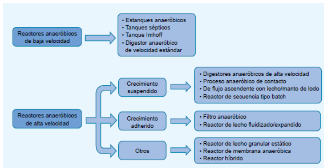
Figura 25. Clasificación de los biorreactores según su velocidad de trabajo. Fuente: Varnero, 2011.
