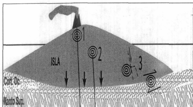
Fig. 8.—Esquema que ilustra los procesos que originan los principales tipos de terremotos en islas volcánicas oceánicas. 1: Fracturación hidráulica, explosivos, «tremor volcánico». 2: Fracturación hidráulica. 3: Fallas normales de asentamiento o inversas de «escape».
