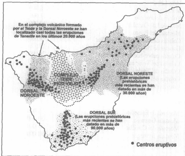
Fig. 3.—Sistema de dorsales y edificio central de Tenerife. Sólo la dorsal noroeste y el edificio central han tenido actividad eruptiva importante en los últimos 30.000 años.
