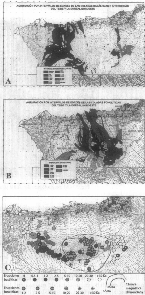
Fig. 6.—Agrupación de las erupciones del Teide y las dorsales NO y NE por edad y composición. A) Coladas basálticas e intermedias. B) Coladas fonolíticas. C) Agrupación de los centros de emisión en función de su composición y edad. Observar la progresiva reducción de la cámara magmática fonolítica del Teide (líneas de trazos), como se deduce del progresivo agrupamiento de los centros de emisión, y la concentración de las basálticas e intermedias en la Dorsal Noroeste.
