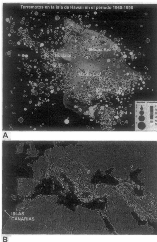
Fig. 7.—A) Terremotos de magnitud >3 registrados en la isla de Hawái en el período 1960-1996. La mayoría son de 5-6 grados de magnitud, pero se han superado los 7. Como puede observarse son todos volcánicos, relacionados con los volcanes activos, incluyendo los de los flancos submarinos, como el volcán submarino Loihi, la próxima isla que emergerá. B) Sismicidad ( M > 5 ) registrada en el Atlántico Norte, Europa y el norte de África en el período 1960-2003. Obsérvese la escasa incidencia en las Islas Canarias, archipiélago volcánico oceánico situado en el interior de la Placa Africana, en comparación con las zonas circundantes de borde de placa (Imágenes tomadas de Earthquakes and Eruptions, de la Smithsonian Institution Global Volcanism Program, www.volcano.si.edu/gvp/ ).
